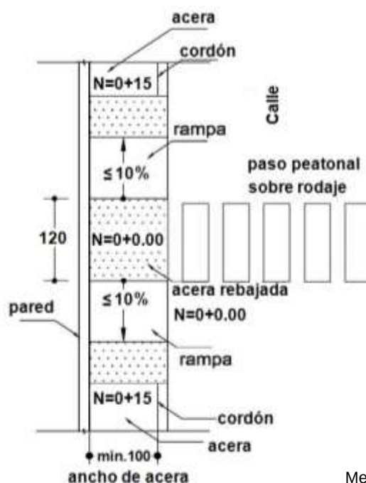
Figura 23 - Vista superior de una acera con dos superficies inclinadas que comienzan desde una superficie a nivel con el rodaje, subiendo en el sentido longitudinal y en todo el ancho de la acera. Se indican los sectores que deberán tener piso táctil de alerta
