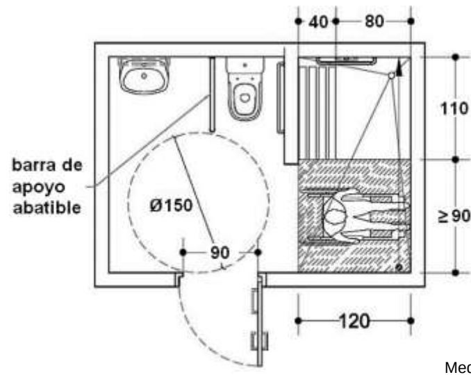
Figura 62 - Vista en planta de un ejemplo de cubículo de baño con su ducha, indicando las medidas respectivas
