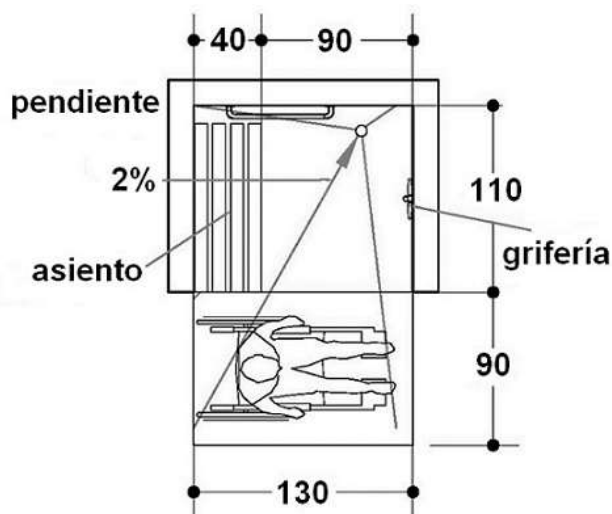
Figura 60 - Vista en planta de una persona usuaria de silla de rueda ubicada de forma lateral a un asiento y a un espacio rectangular que indica el espacio de una ducha con su respectiva barra de apoyo y grifería
