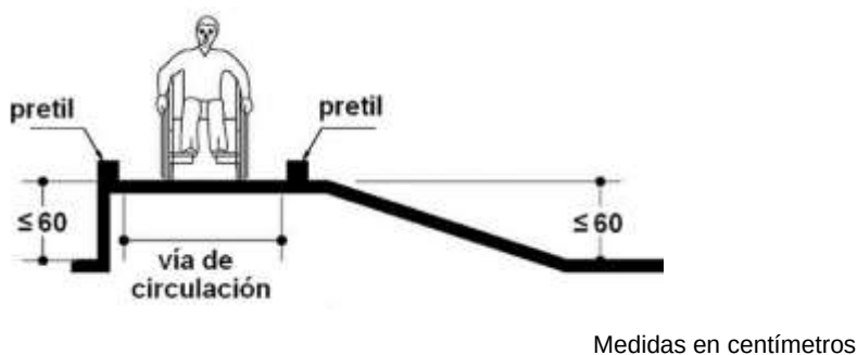
Figura 31 - Vista en elevación frontal de vía de circulación: describe un desnivel respecto a la superficie adyacente entre 18 cm y 60 cm donde se interpone una zona de seguridad de 60 cm de ancho y una rampa que conecta ambas superficies
