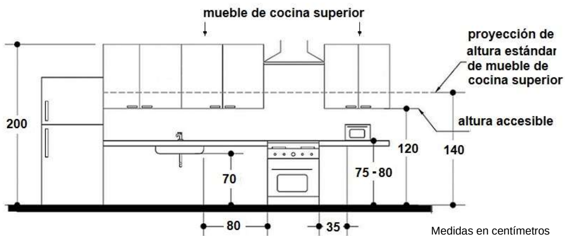
Figura 50 - Vista en elevación frontal del espacio de una cocina con superficies de apoyo a ambos lados, con su lavatrastos en el centro, una refrigeradora, así como un mueble de cocina en la parte superior
